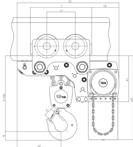
Model Yalelift LHG, 10.000 kg, üçlü
