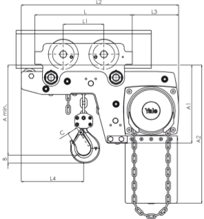
Model Yalelift LHG, 500 - 3.000 kg, tekli
